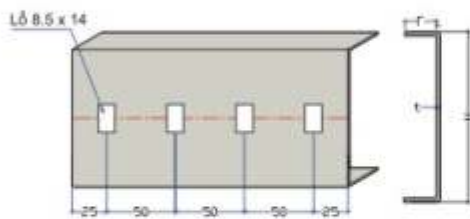
NỐI THẰNG THANG CÁP
