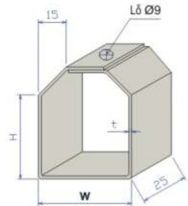
TREO MÁNG CÁP
