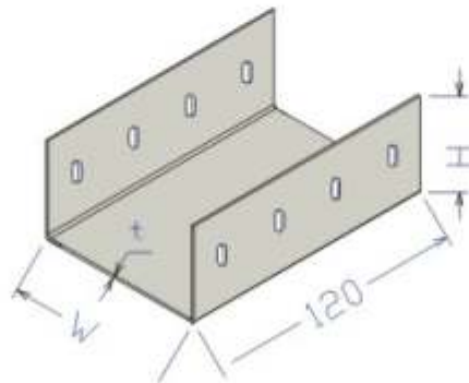
NỐI THẲNG MÁNG CÁP
